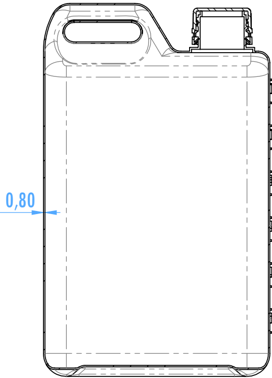
SECCIÓN C-C
