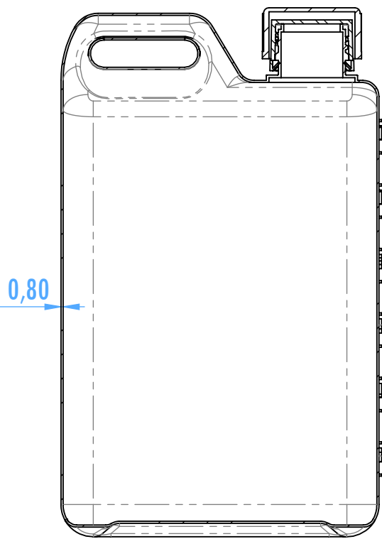
SECCIÓN F-F
