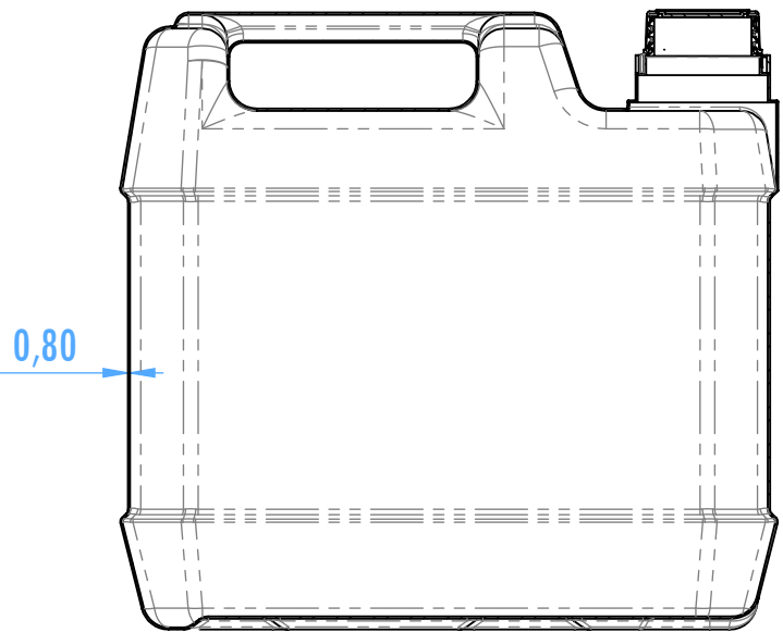
SECCIÓN I-I
