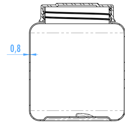
SECCIÓN E-E
