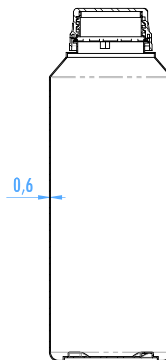
SECCIÓN E-E
