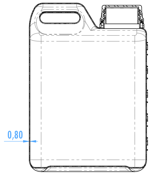
SECCIÓN E-E
